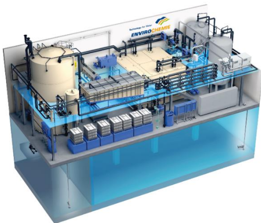
Bild: Entfernung von aktiven Wirkstoffen aus dem Abwasser einer Pharmaproduktion.
