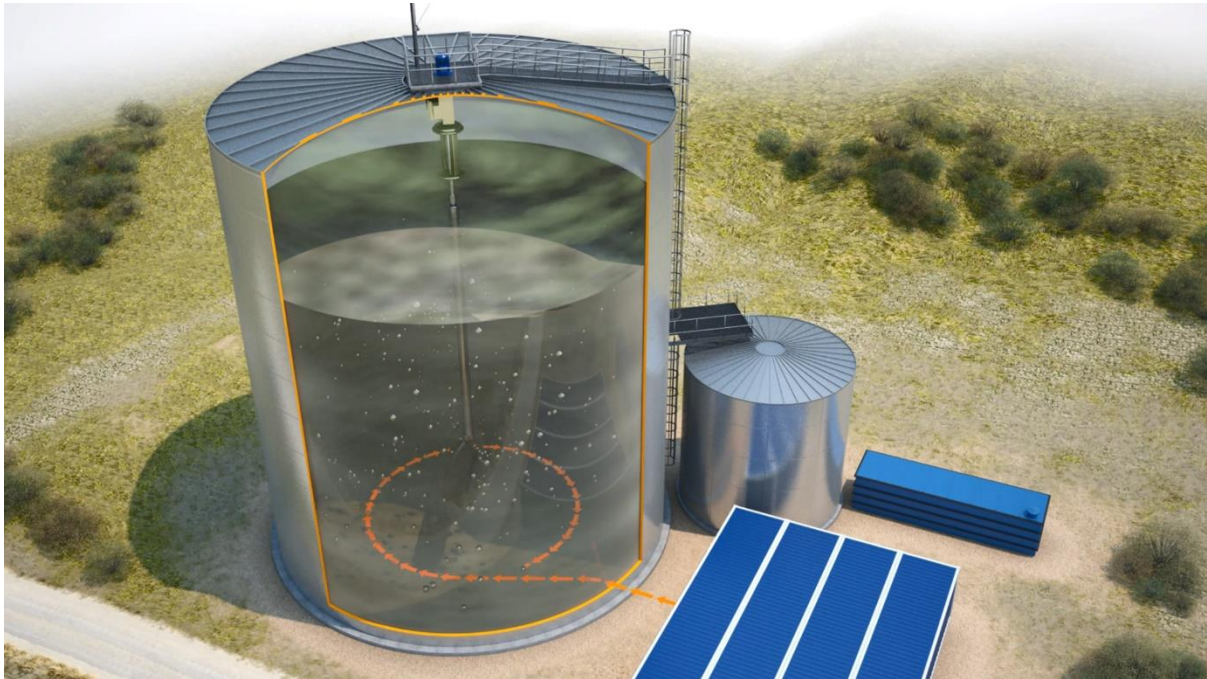
Im Anaerobreaktor Biomar AWR werden hochbelastete Abwässer und Flüssigabfälle in Biogas umgewandelt
