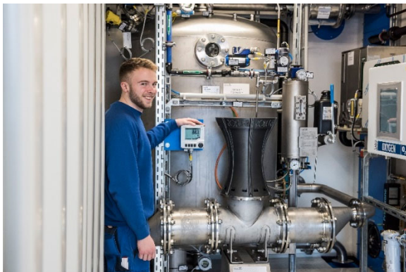
AOP mittels Ozon mit einem Roturi zur sicheren Entfernung von Medikamentenspuren aus dem Abwasser
